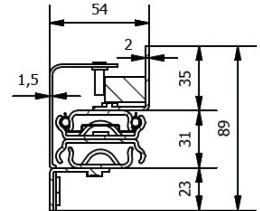
A-A (1:3)
