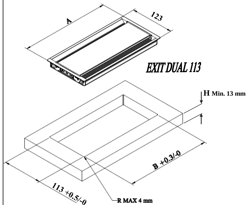
DIMENSIONI TAGLIO PIANO(mm) TABLE CUTTING DIMENSIONS(mm)
